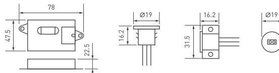
Рисунок 1. Габаритные размеры ИК-датчика SR-PRIME
