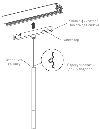
Рис. 2. Установка светильника
