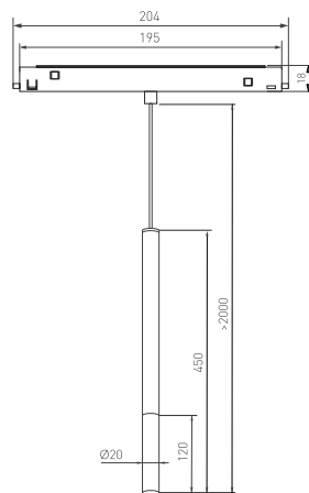
Рис. 1. Чертеж и габаритные размеры
