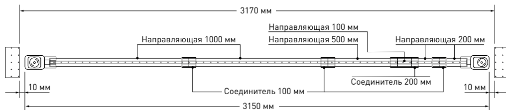
Рис. 4. Пример сборки направляющей длиной 3.15 м
