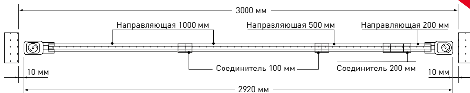
Рис. 3. Пример сборки направляющей длиной 2.92 м
