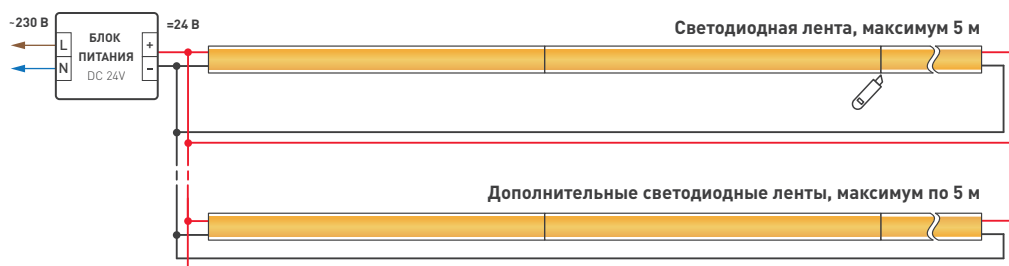
Схема 1. Подключение нескольких светодиодных лент с двух сторон. Использовать для обеспечения равномерного свечения ленты по всей длине.
